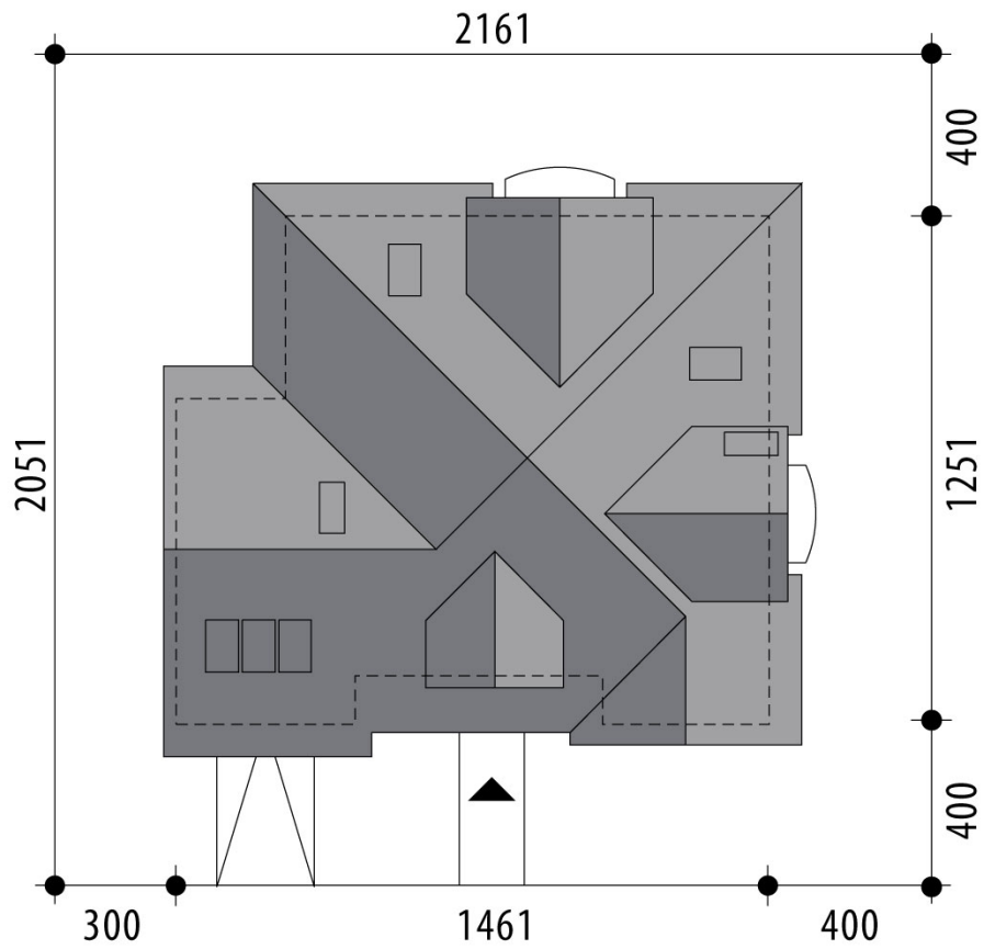
RZUT DZIAŁKI
