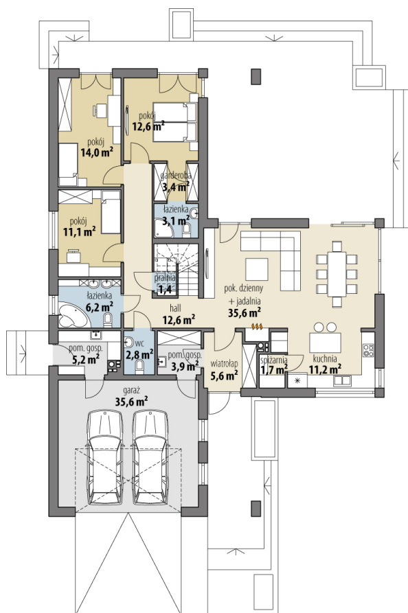
RZUT PARTER
