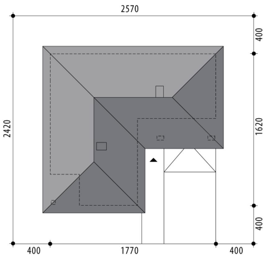
RZUT DZIAŁKI
