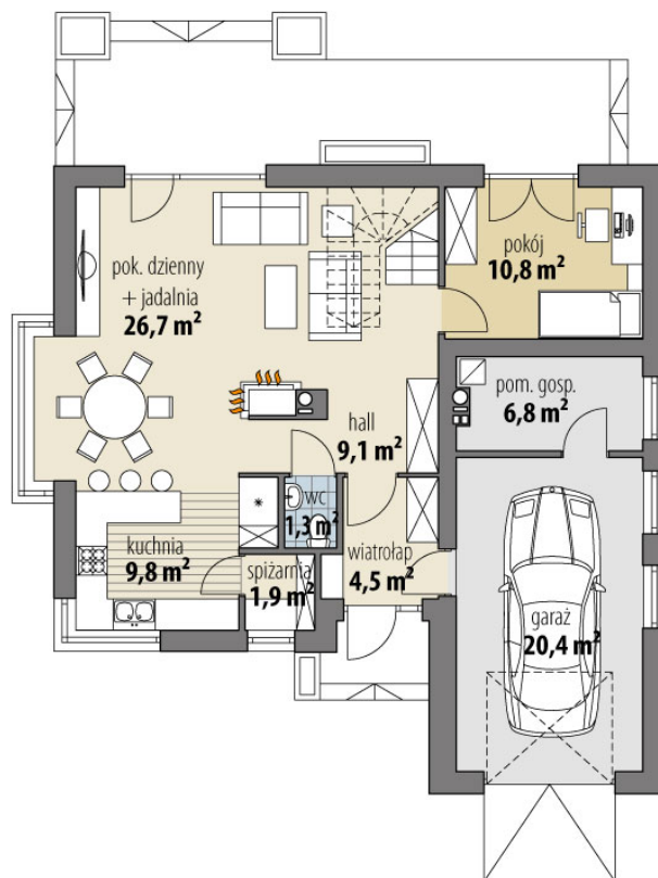
RZUT PARTER
