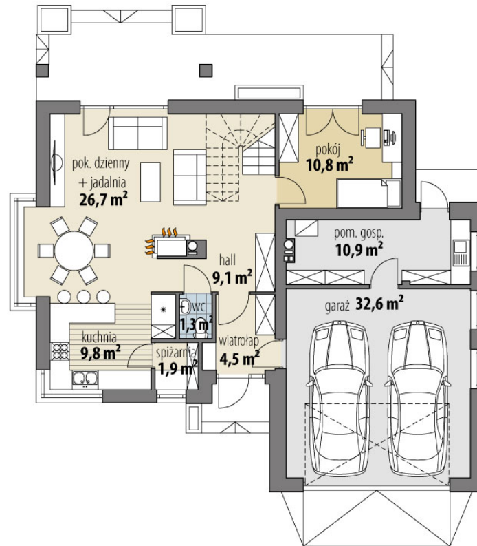
RZUT PARTER
