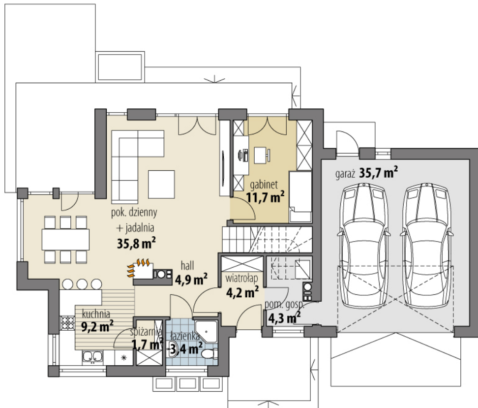
RZUT PARTER
