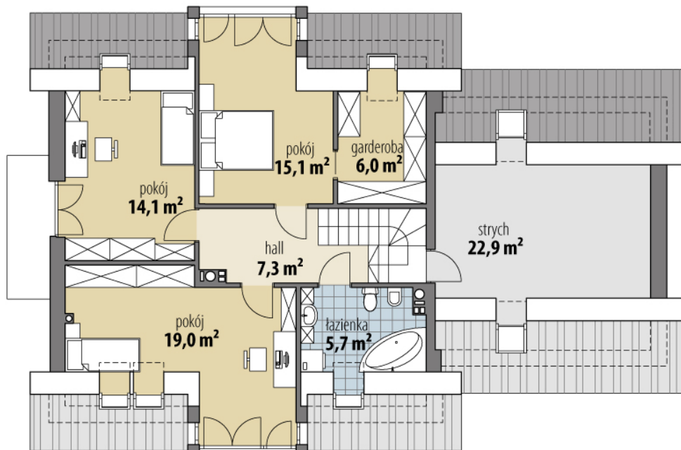
RZUT
