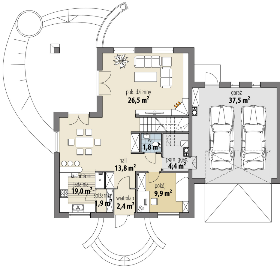
RZUT PARTER
