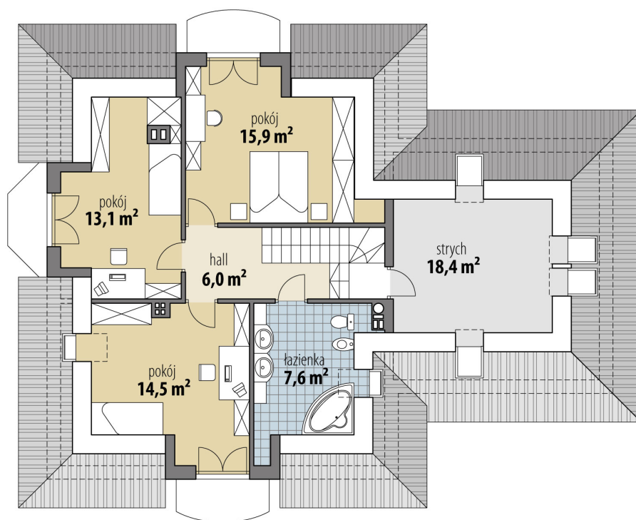
RZUT
