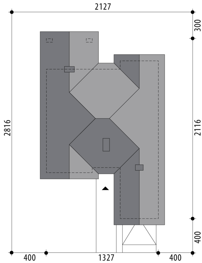
RZUT DZIAŁKI
