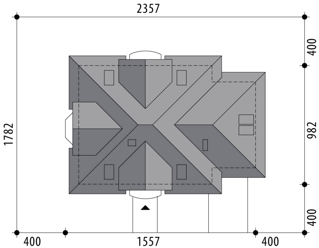
RZUT DZIAŁKI
