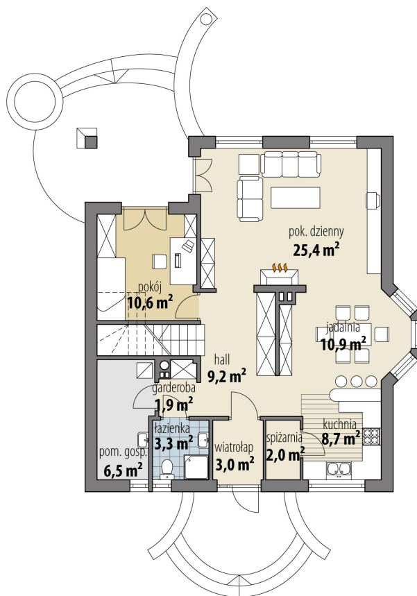
RZUT PARTER
