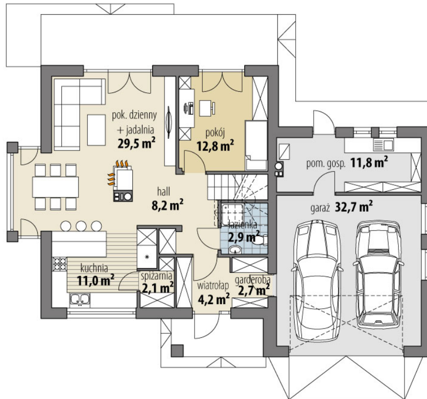
RZUT PARTER
