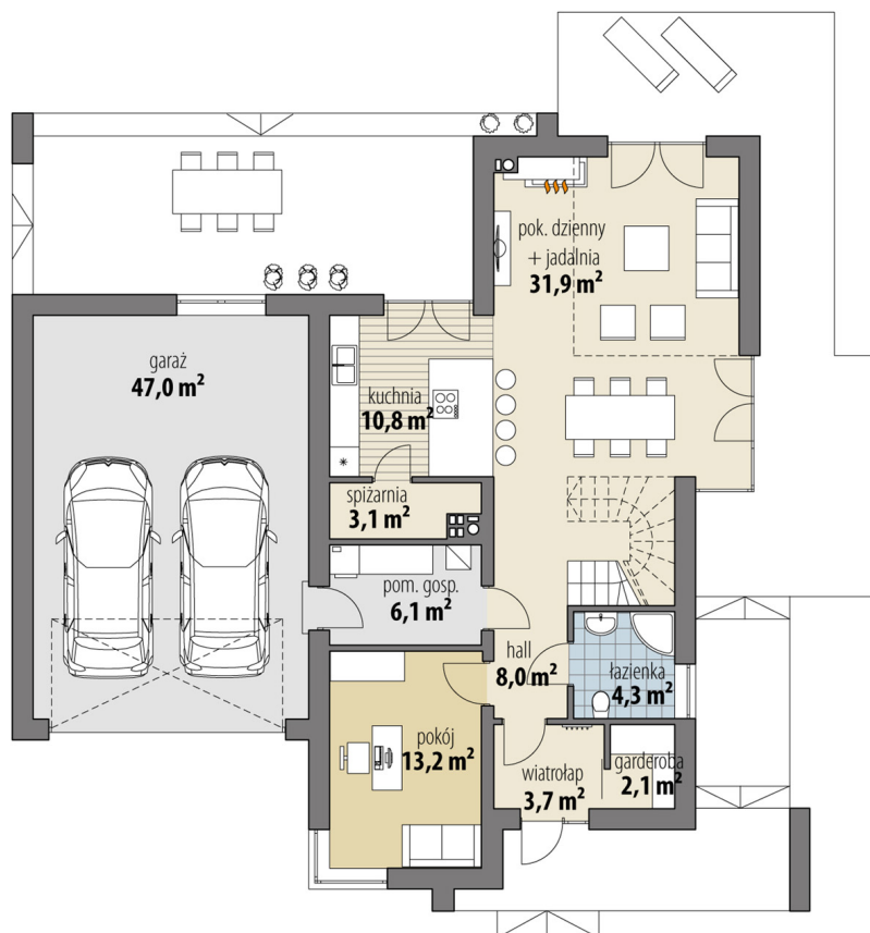
RZUT PARTER
