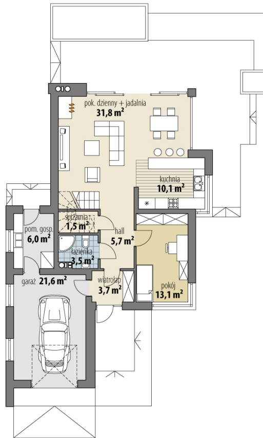
RZUT PARTER
