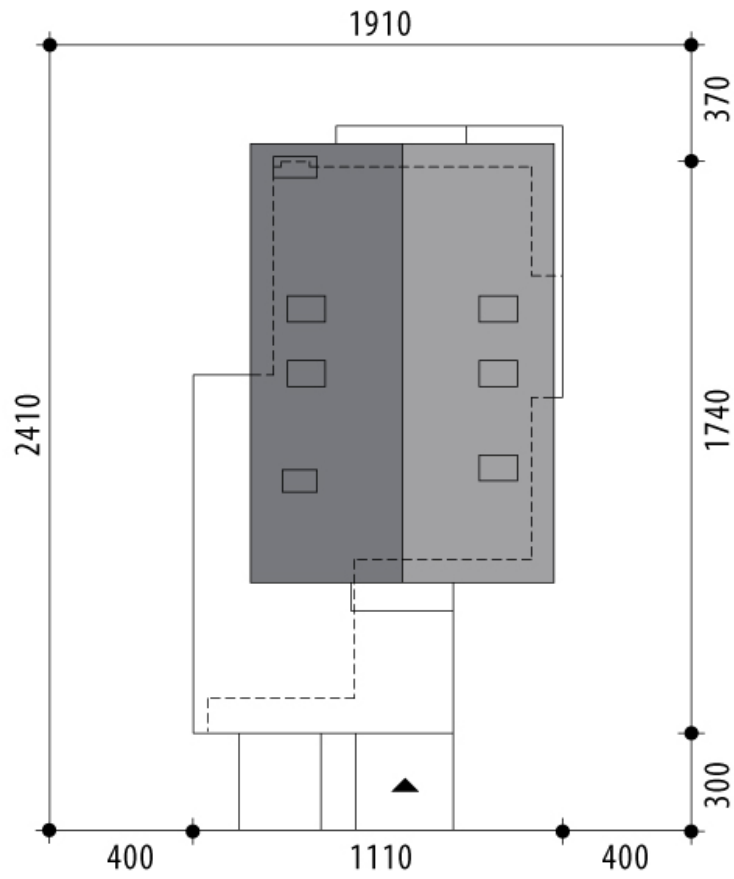
RZUT DZIAŁKI
