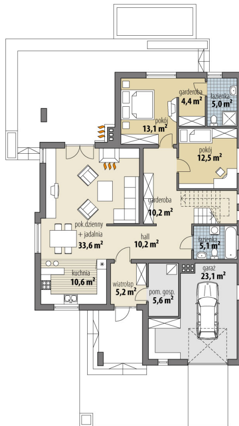
RZUT PARTER
