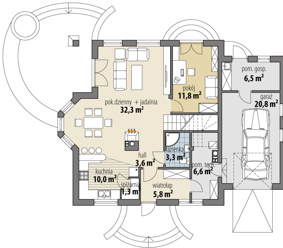
RZUT PARTER
