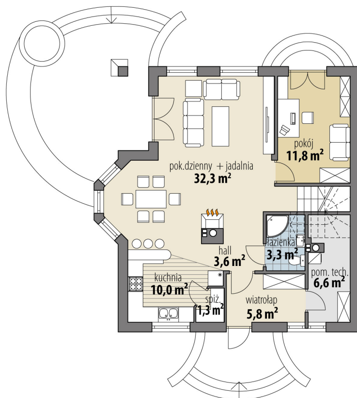
RZUT PARTER
