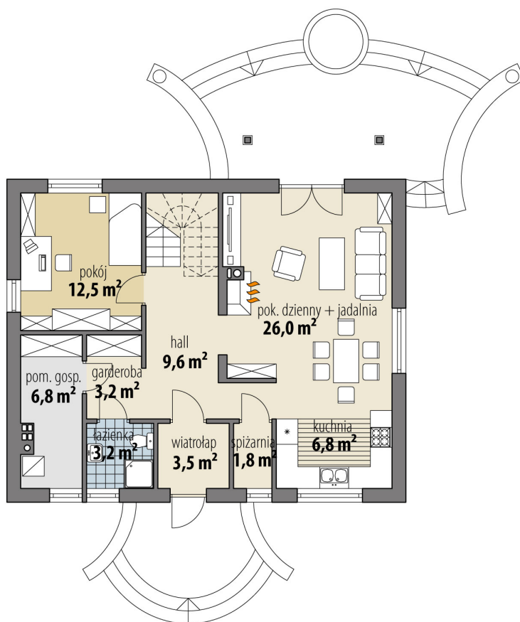
RZUT PARTER
