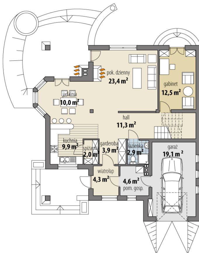
RZUT PARTER
