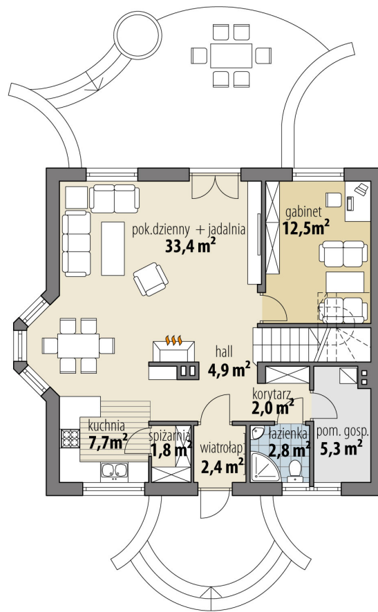
RZUT PARTER
