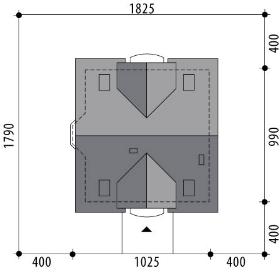
RZUT DZIAŁKI
