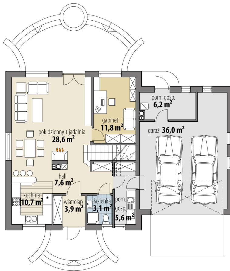
RZUT PARTER
