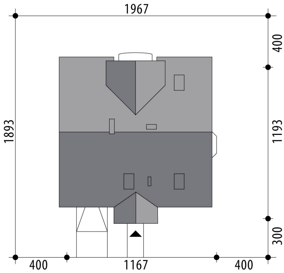
RZUT DZIAŁKI
