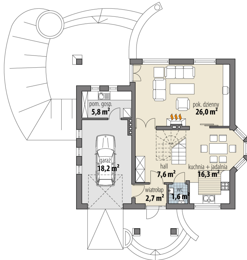
RZUT PARTER
