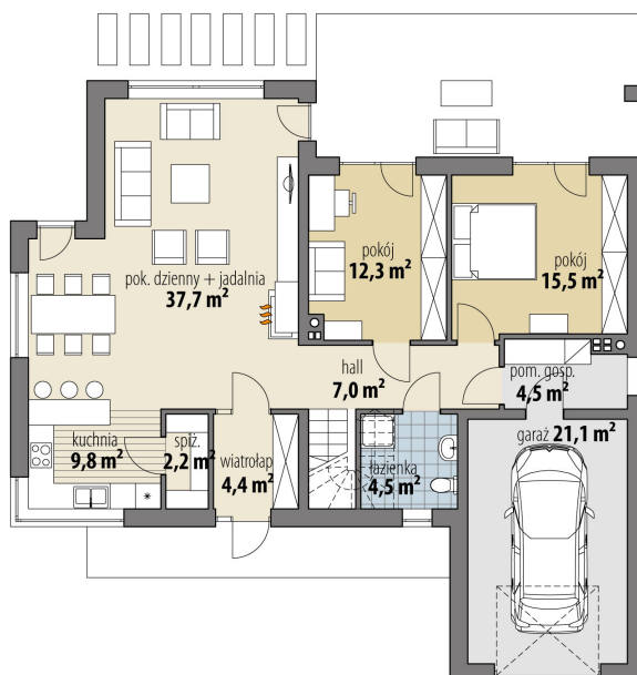
RZUT PARTER
