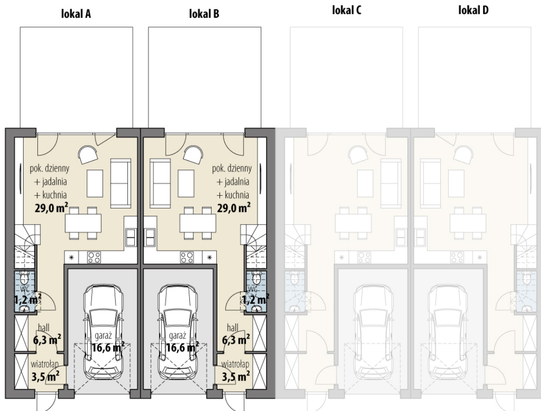
RZUT PARTER
