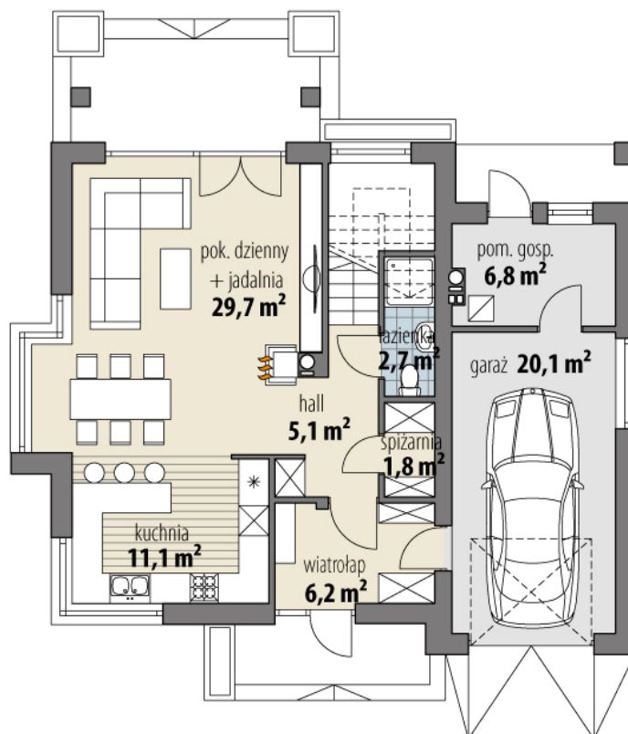
RZUT PARTER
