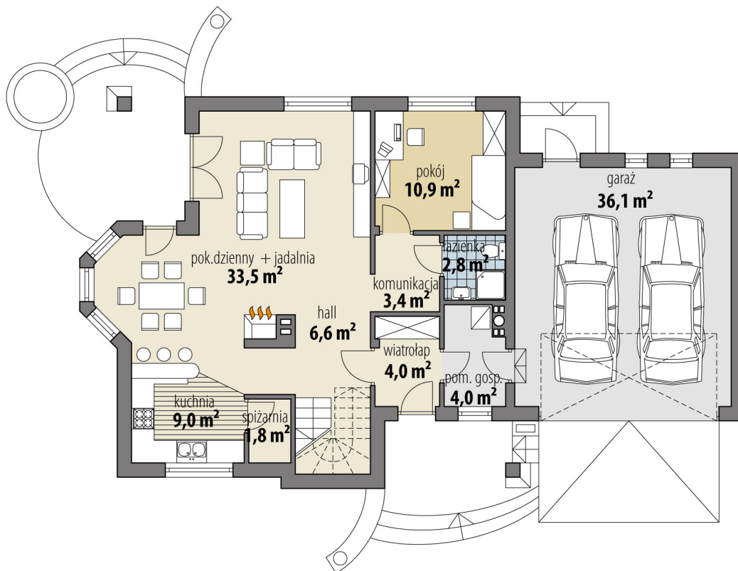
RZUT PARTER
