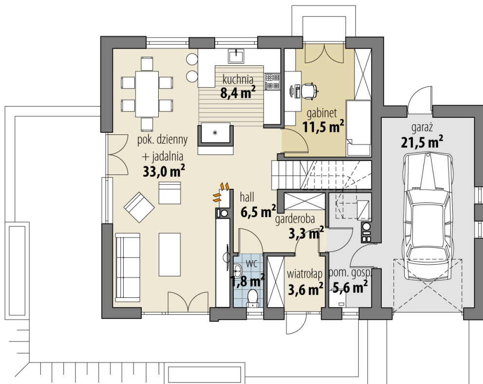
RZUT PARTER
