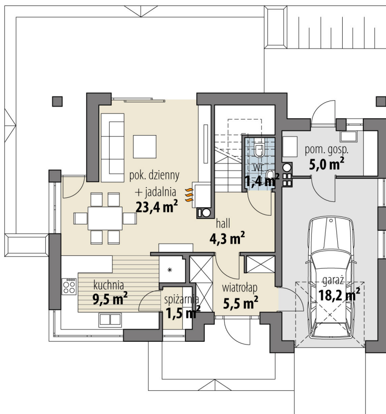
RZUT PARTER
