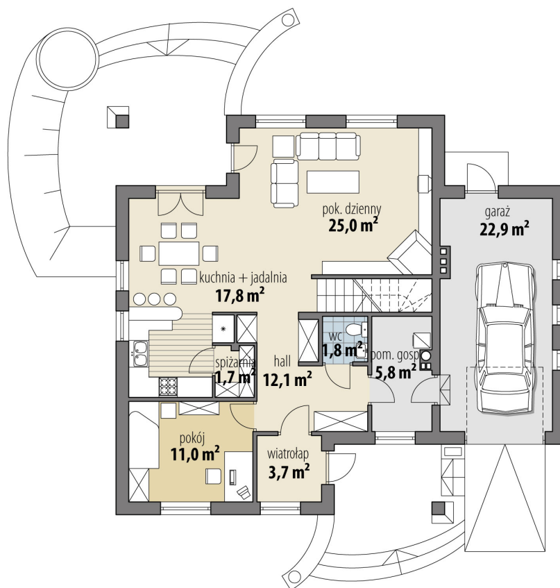
RZUT PARTER
