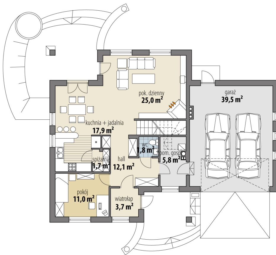
RZUT PARTER
