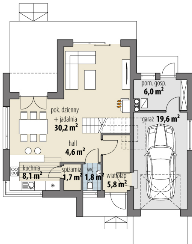
RZUT PARTER
