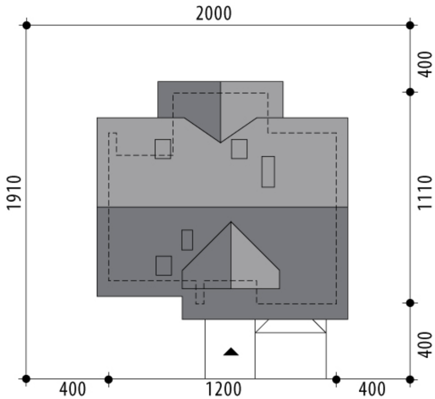
RZUT DZIAŁKI
