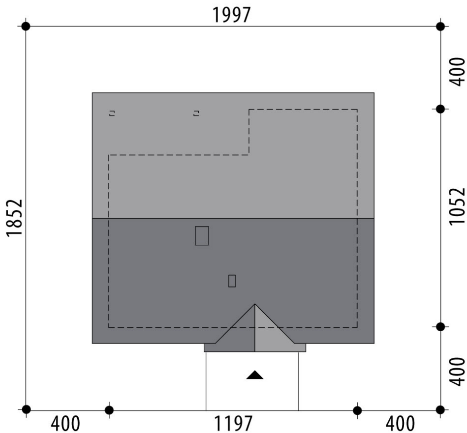
RZUT DZIAŁKI
