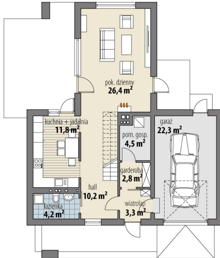
RZUT PARTER
