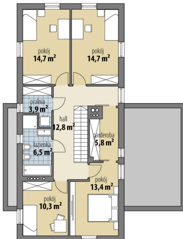
RZUT
