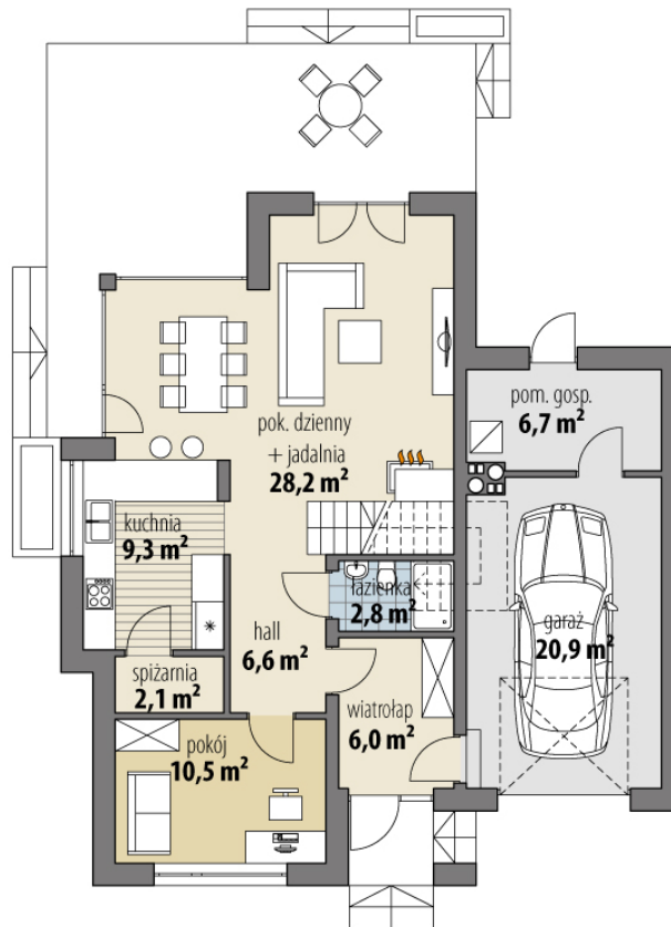
RZUT PARTER
