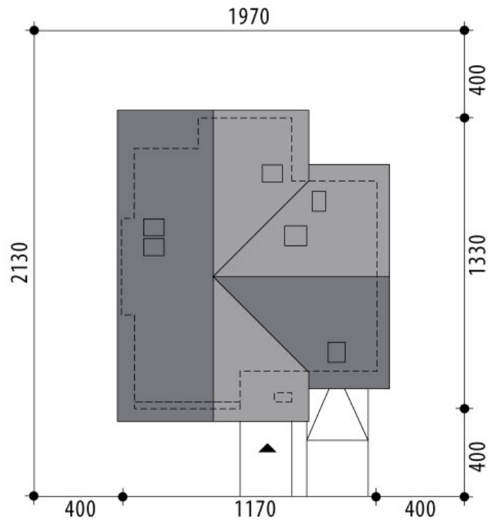
RZUT DZIAŁKI
