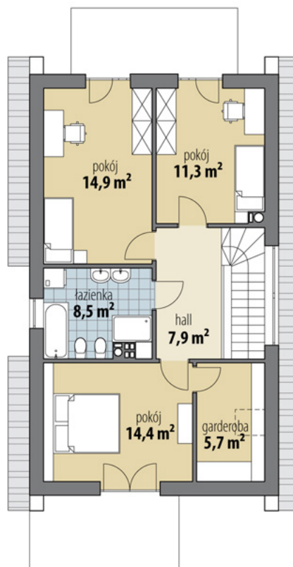
RZUT
