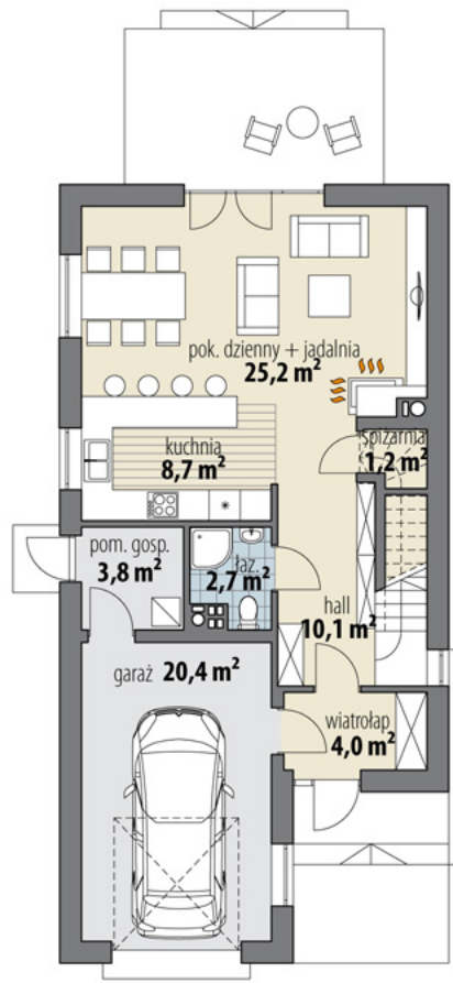
RZUT PARTER
