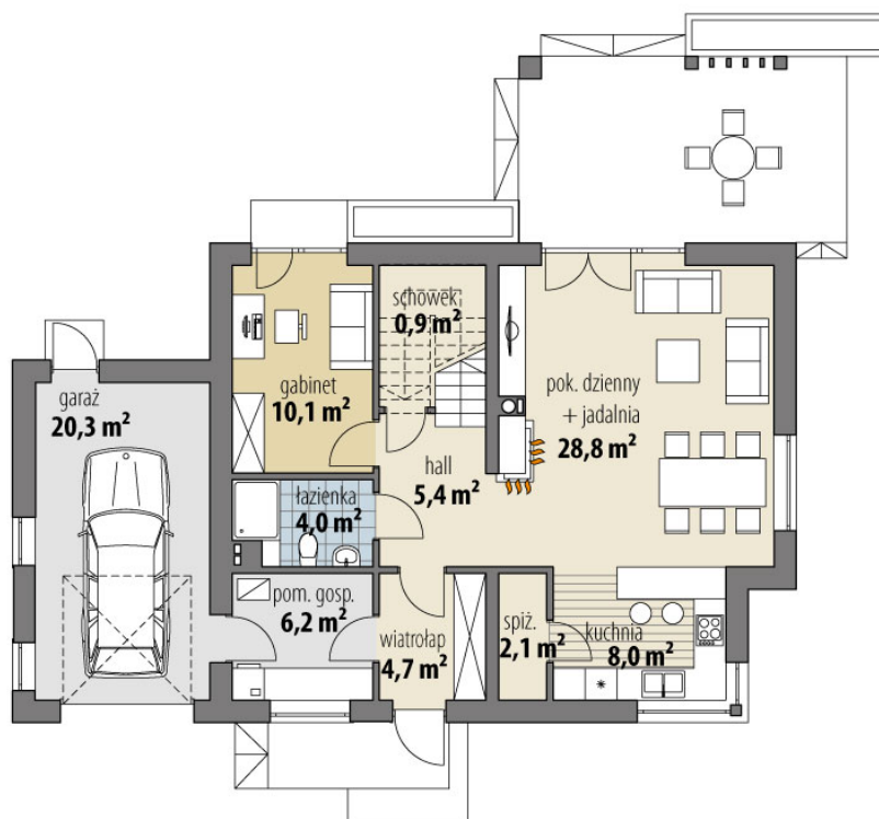
RZUT PARTER
