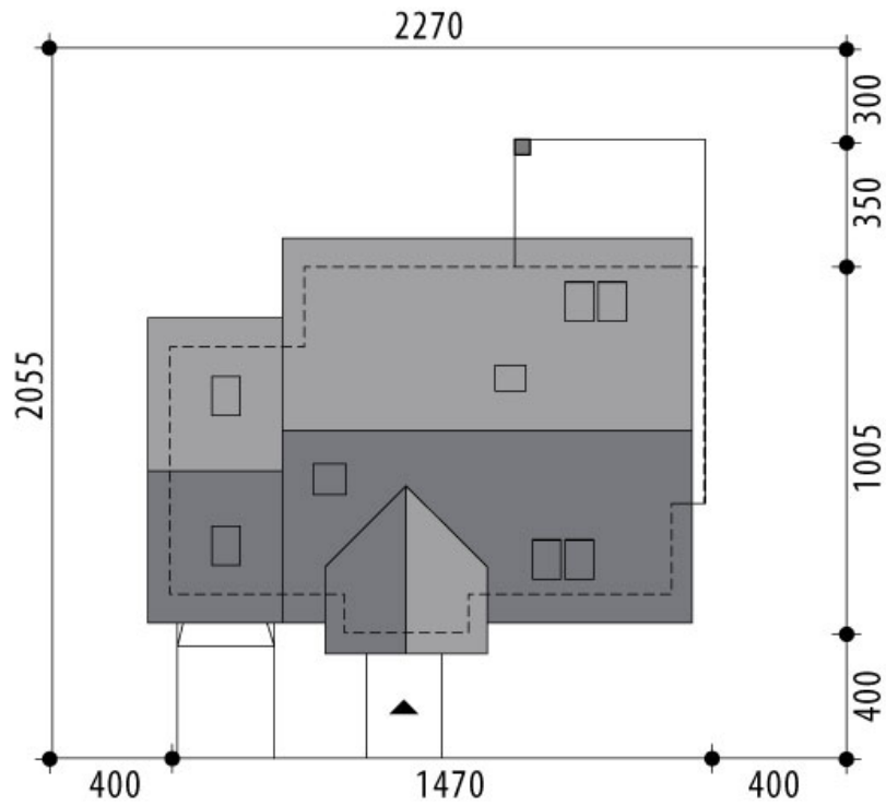
RZUT DZIAŁKI
