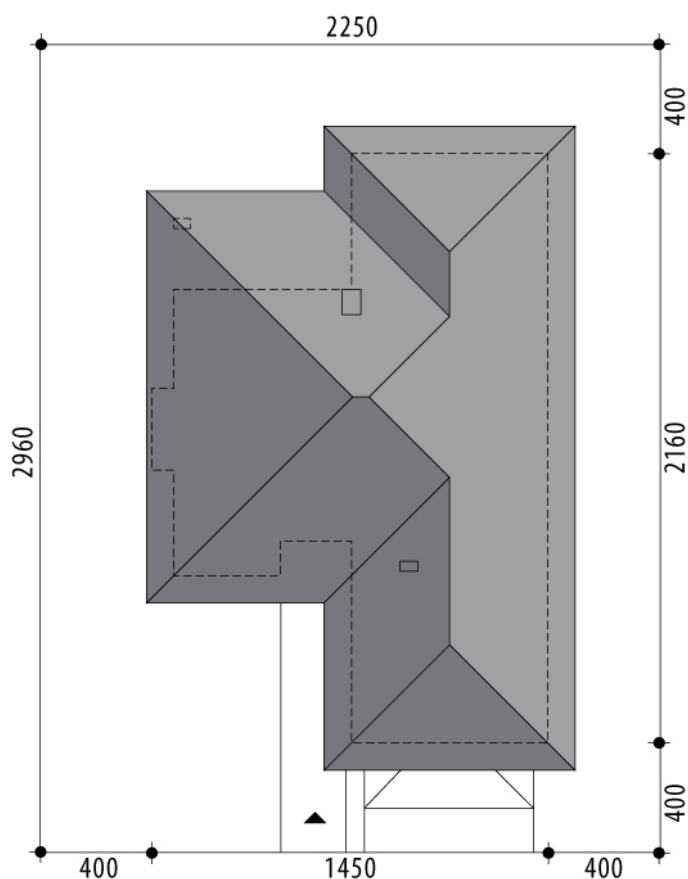
RZUT DZIAŁKI
