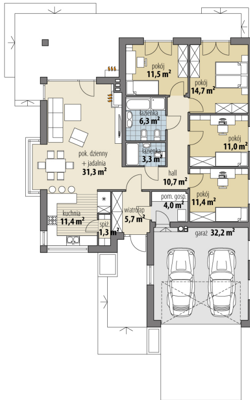
RZUT PARTER
