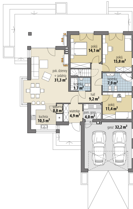
RZUT PARTER
