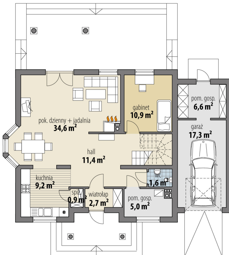
RZUT PARTER
