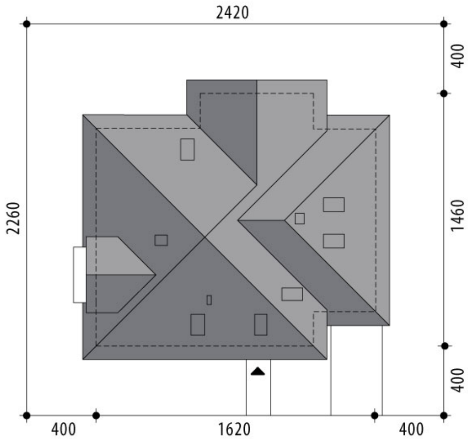
RZUT DZIAŁKI
