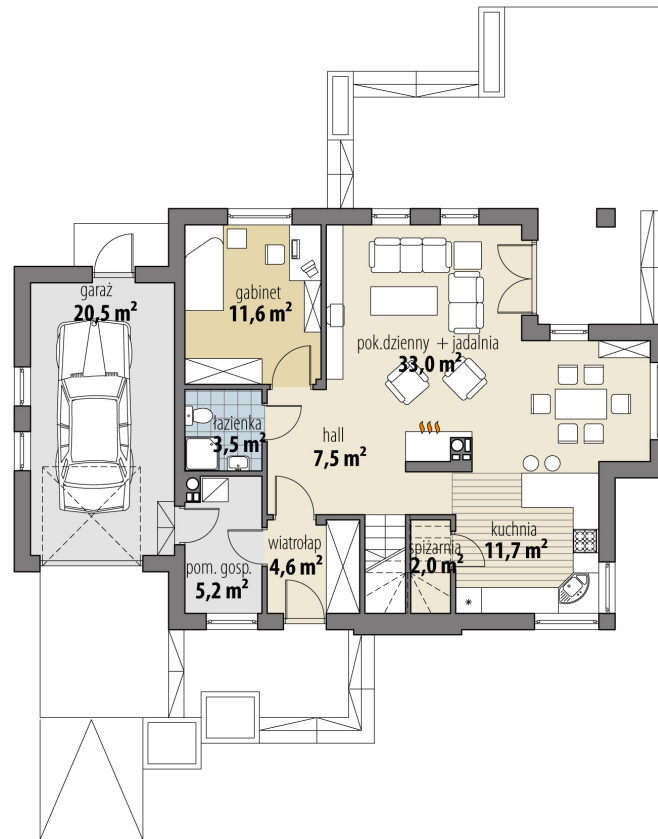
RZUT PARTER
