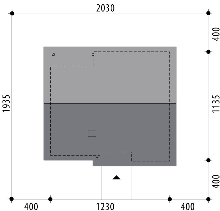
RZUT DZIAŁKI
