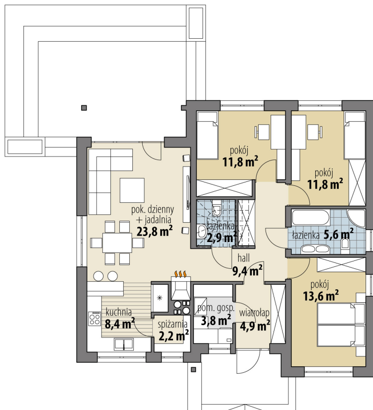
RZUT PARTER
