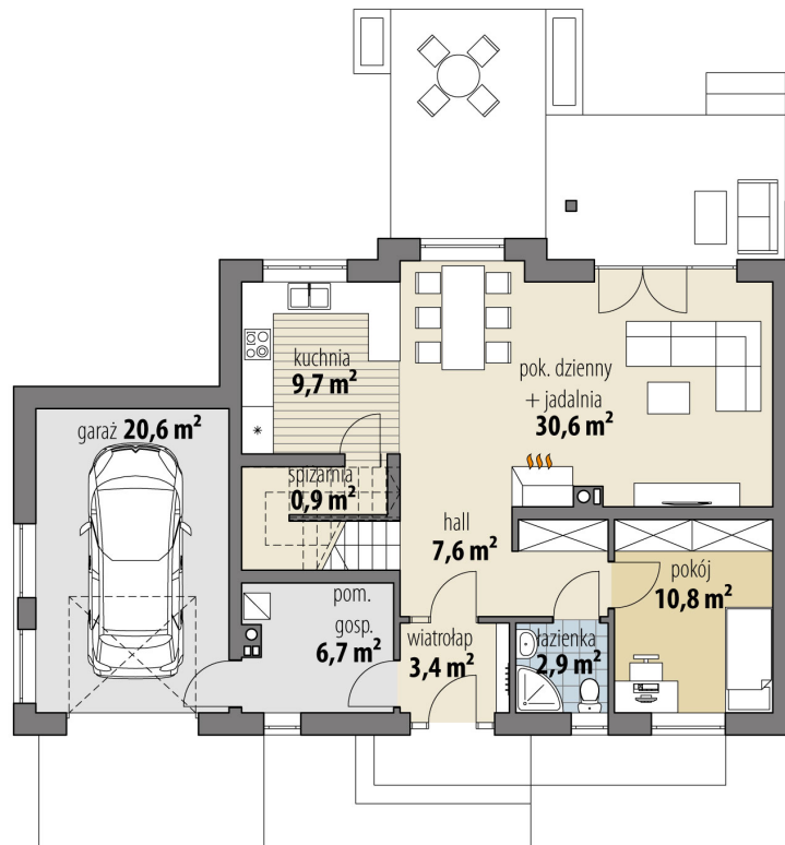
RZUT PARTER
