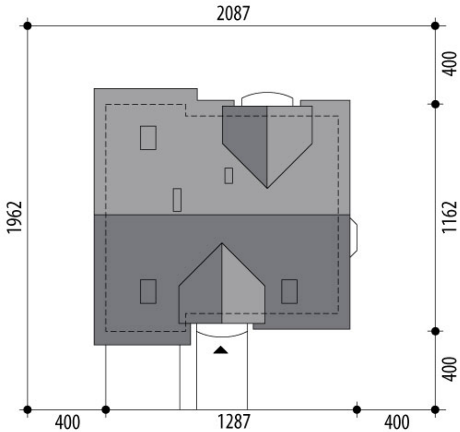
RZUT DZIAŁKI
