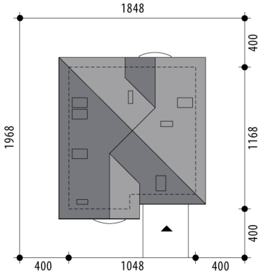
RZUT DZIAŁKI
