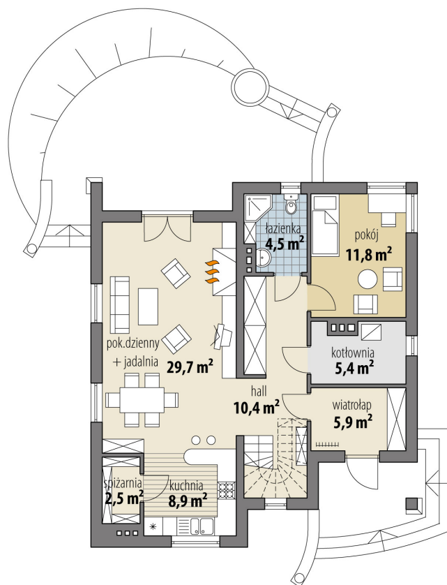
RZUT PARTER
