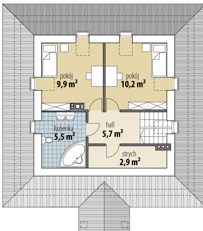
RZUT
