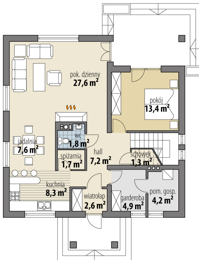
RZUT PARTER
