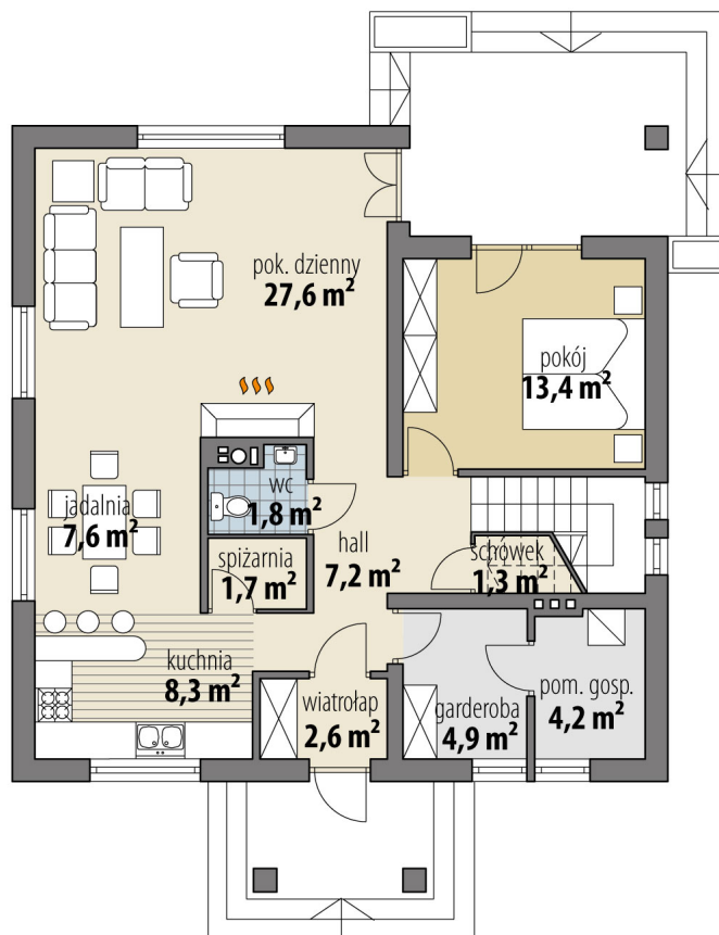
RZUT PARTER
