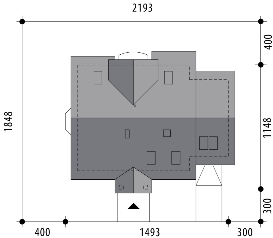
RZUT DZIAŁKI
